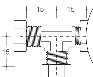
Modello / Model: AR270R
